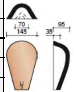
Начальная хребтовая черепица угловая малая
