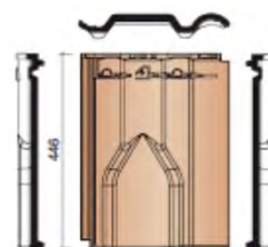
Вентиляционная черепица
