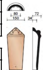
Начальная хребтовая черепица полукруглая
