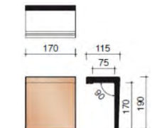
Пультовая моночерепица 90°
