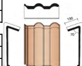
Пультовая моночерепица
