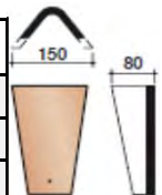
Хребтовая черепица угловая малая
