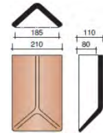
Вальмовая черепица (для хребта bonnet)
