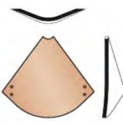
Черепица ендовы 303 35°-50°
