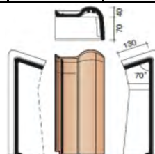
Боковая пультовая моночерепица правая
