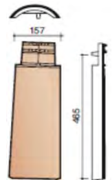
Черепица 1/2
