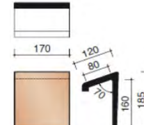
Пультовая моночерепица 70°
